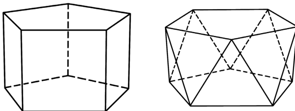
Obr. 1: Pětiboký hranol a antihranol jako polopřávidelná tělesa.
