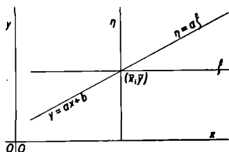
Obr. 12. Rovnice přímky odhadu v původních proměnných a v odchylkách od průměrů.
