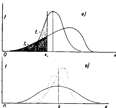
Obr. 2. Množství informace obsažené jen a) v relativní četnosti, b) v průměru.
