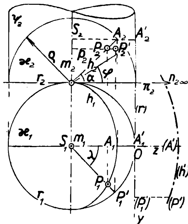
Obr. 48. Stejnoplaché zobrazení kulové plochy na rovinu.
