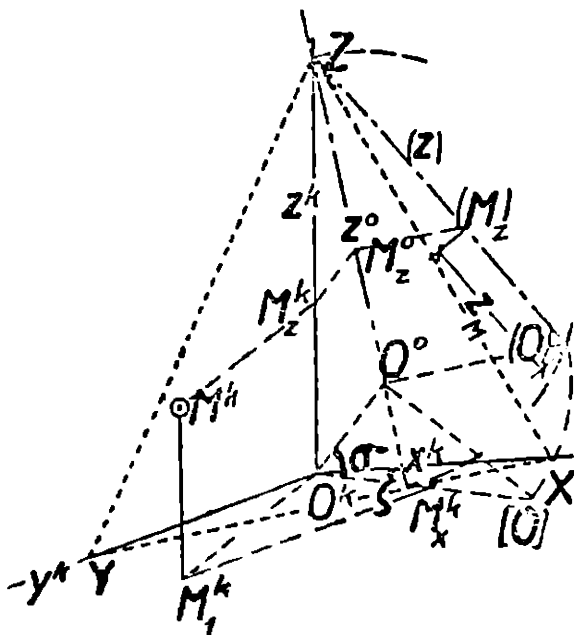
Obr. 34. Kosoúhlá axonometrie. Obrazy bodu M .
