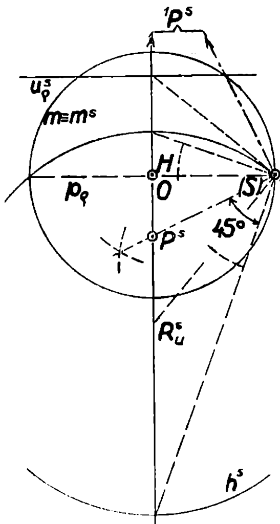
Obr. 14. Stereografický průmět hlavní kružnice kulové plochy.
