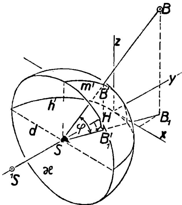
Obr. 17. Základy křivočaré perspektivy. (Stereosférická perspektiva.)
