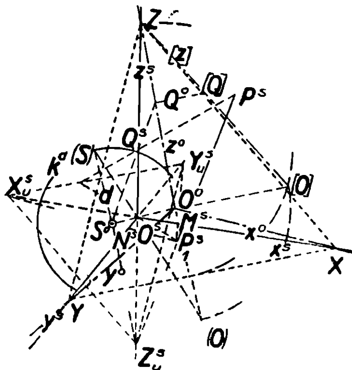
Obr. 38. Středová axonometrie.
