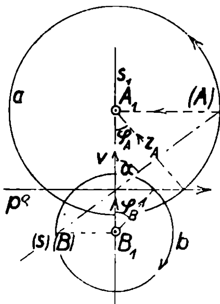
Obr. 52. Cyklografický průmět roviny \varrho .
