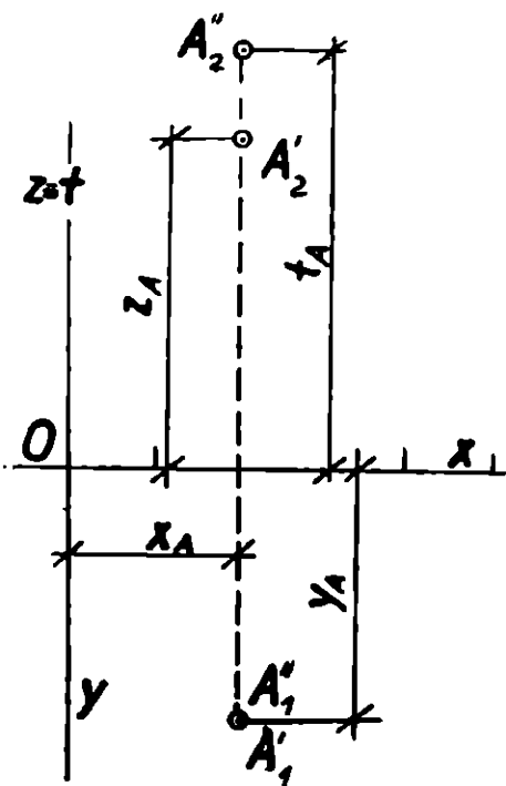
Obr. 55. Zobrazení bodu A čtyřrozměrného prostoru do A_1', A_2', A_3' .
