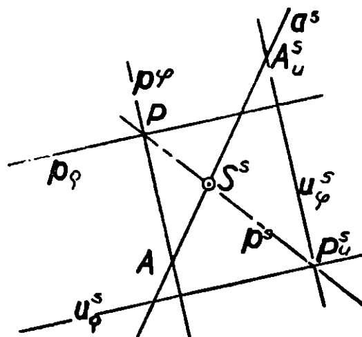
Obr. 6. Průsečík S přímky a s rovinou \rho .
