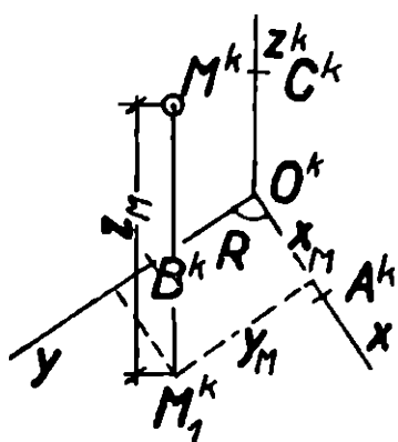
Obr. 37. Vojenská perspektiva bodu M .
