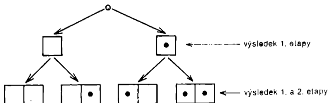
[Obr. 2.5. Strom dvojího hodu s-kostkou
