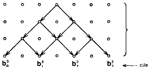
Obr. 6.9. Síť odpovídající třídennímu závodě na šachovnici
